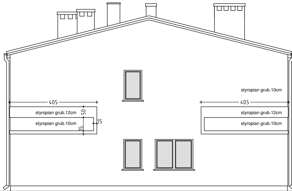
ELEWACJA POŁUDNIOWA
